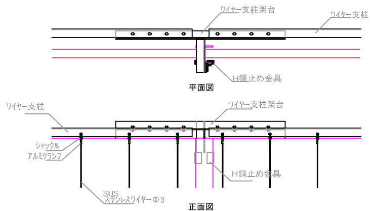
上部拡大図
