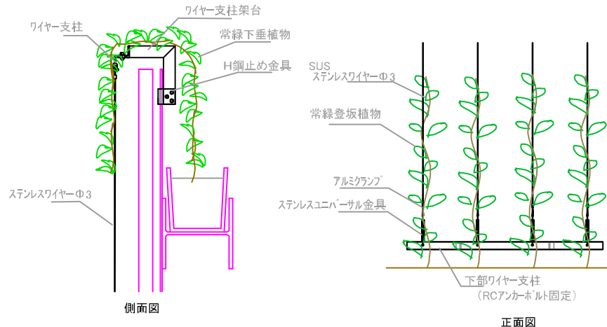
下部拡大図
